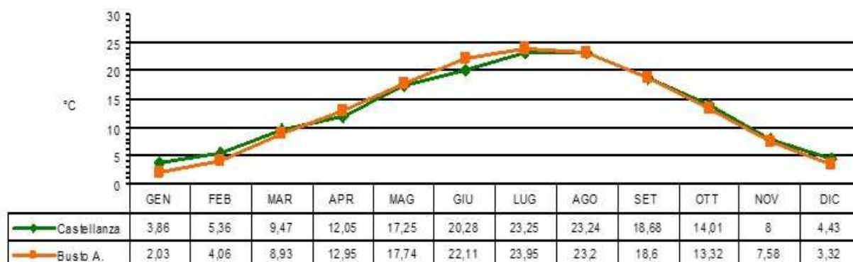
Termogramma; stazioni di CASTELLANZA (VA) e BUSTO A.
