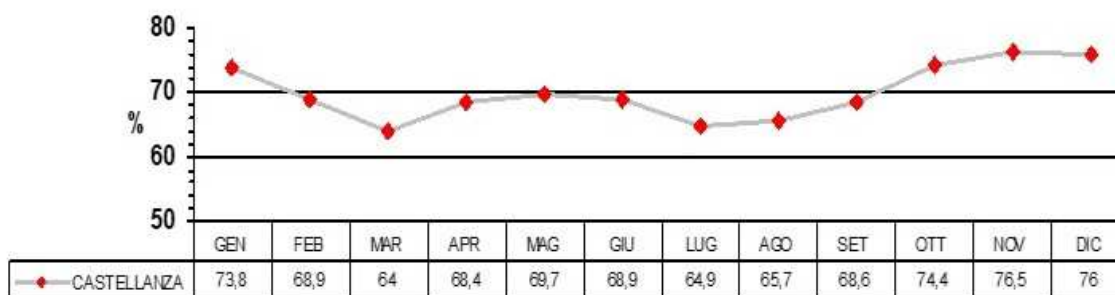
Umidità relativa media; stazione di CASTELLANZA (VA)
