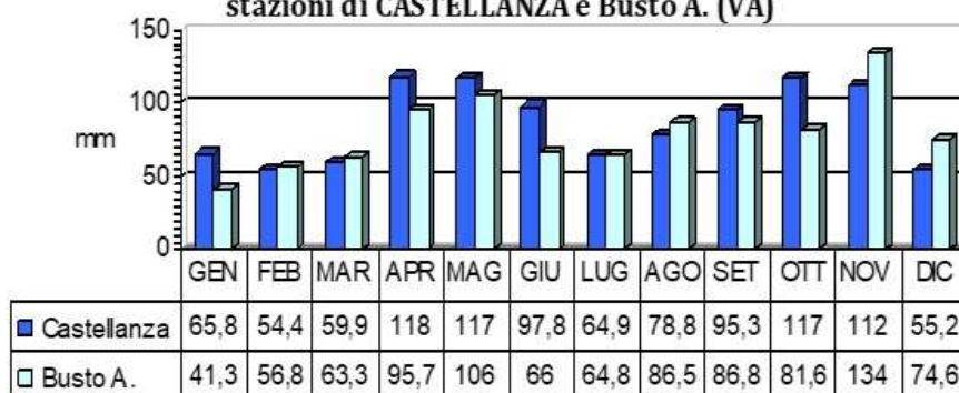
Precipitazioni medie mensili; stazioni di CASTELLANZA e Busto A. (VA)
